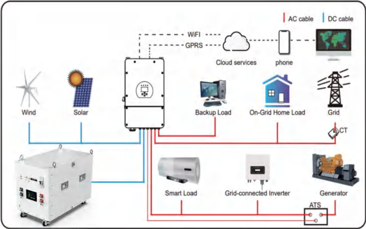
系统连接图System Connection Diagram
